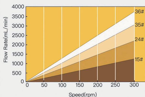
Flow Rate(0.1-350rpm)
